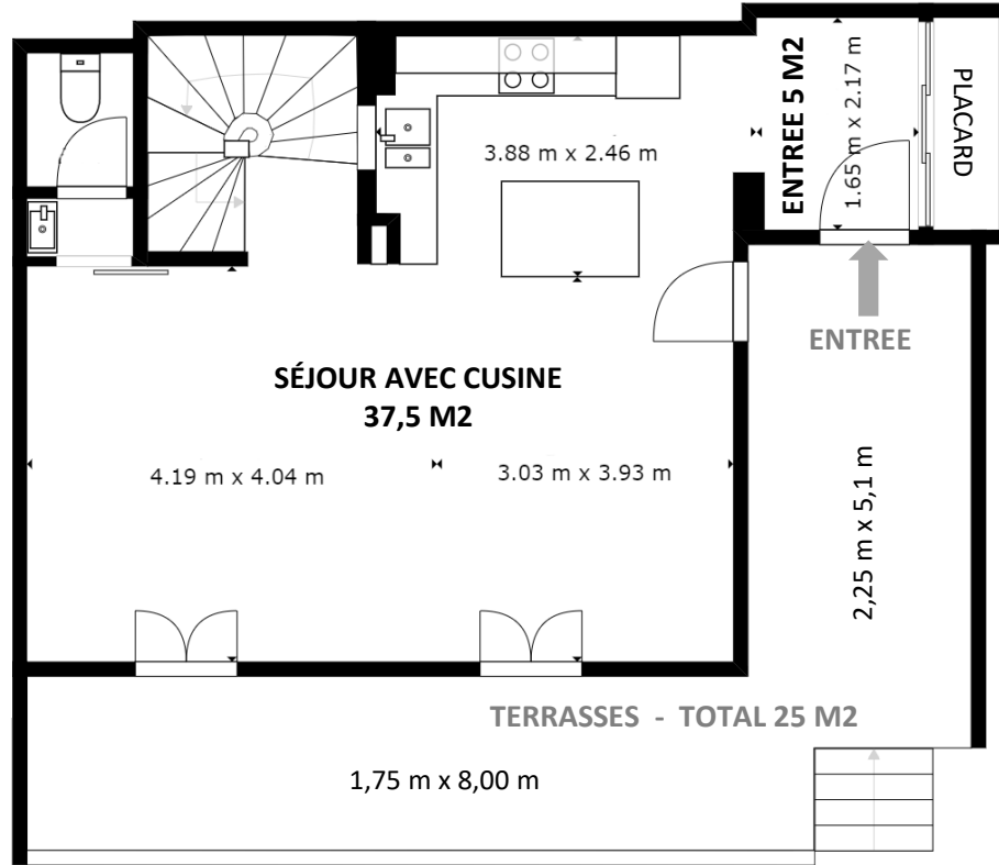
REZ-DE-CHAUSSÉE (Floor2)
